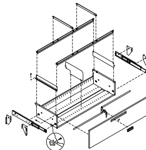
Tiroirs fermés (serrure)
